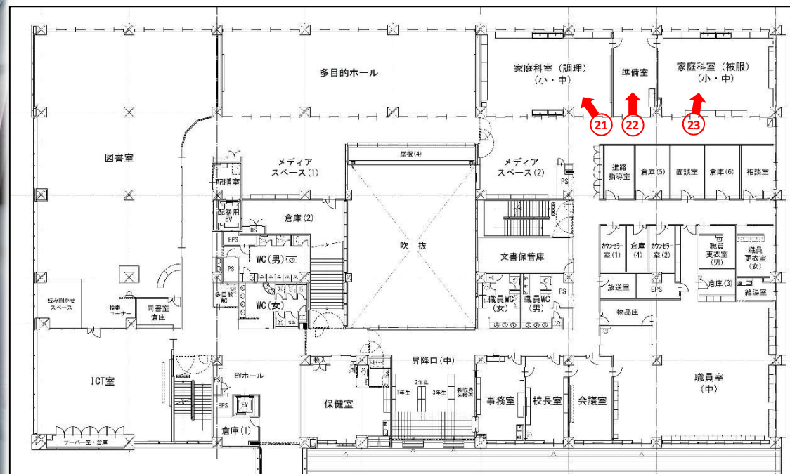
校舎棟 3階平面図
