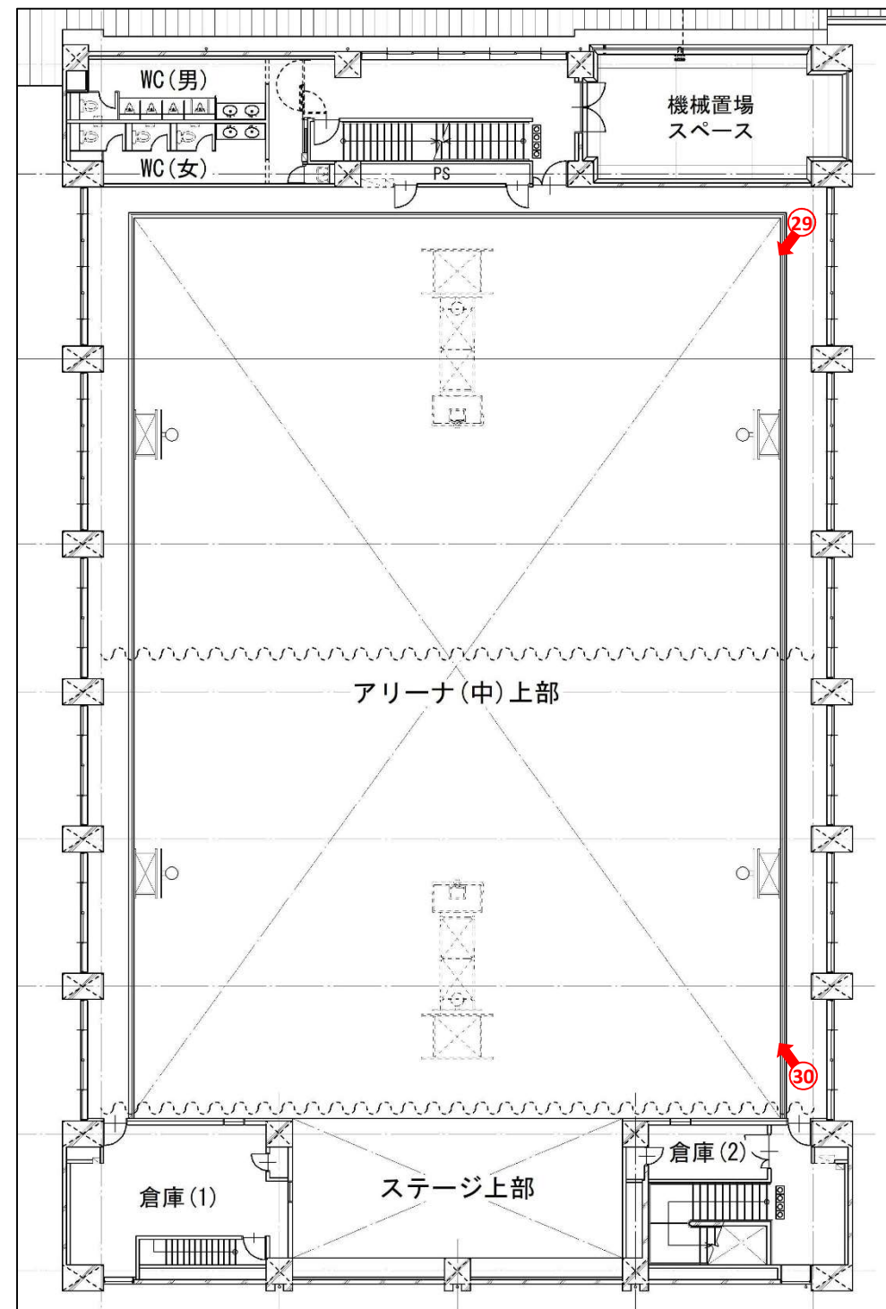
体育館棟 3階平面図
