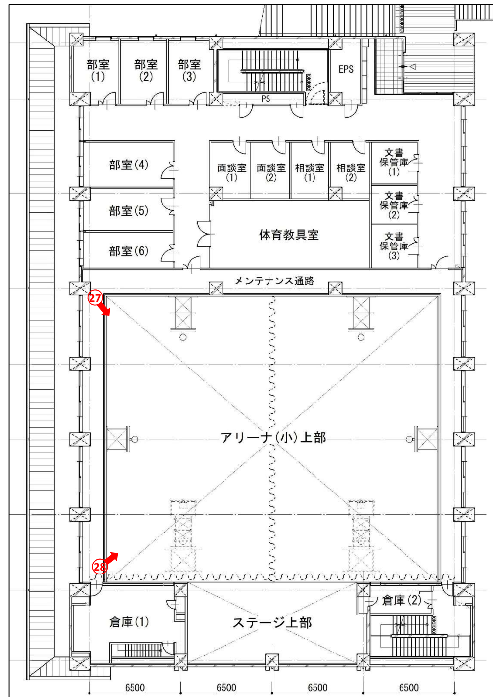
体育館棟 2階平面図
