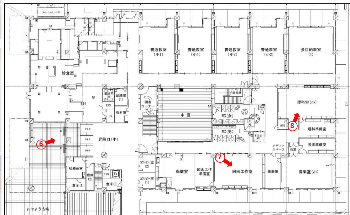
校舎棟 1階平面図
