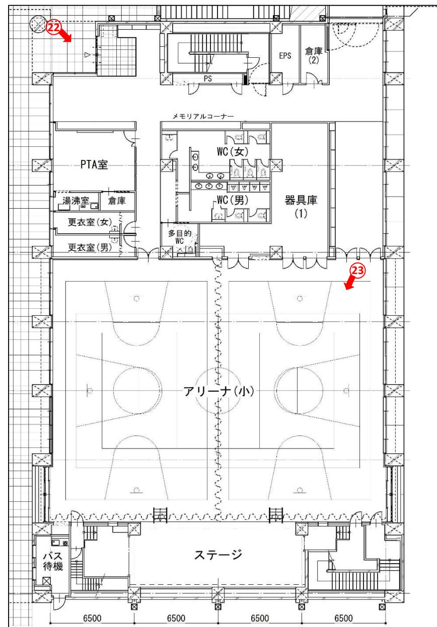
体育館棟 1階平面図
